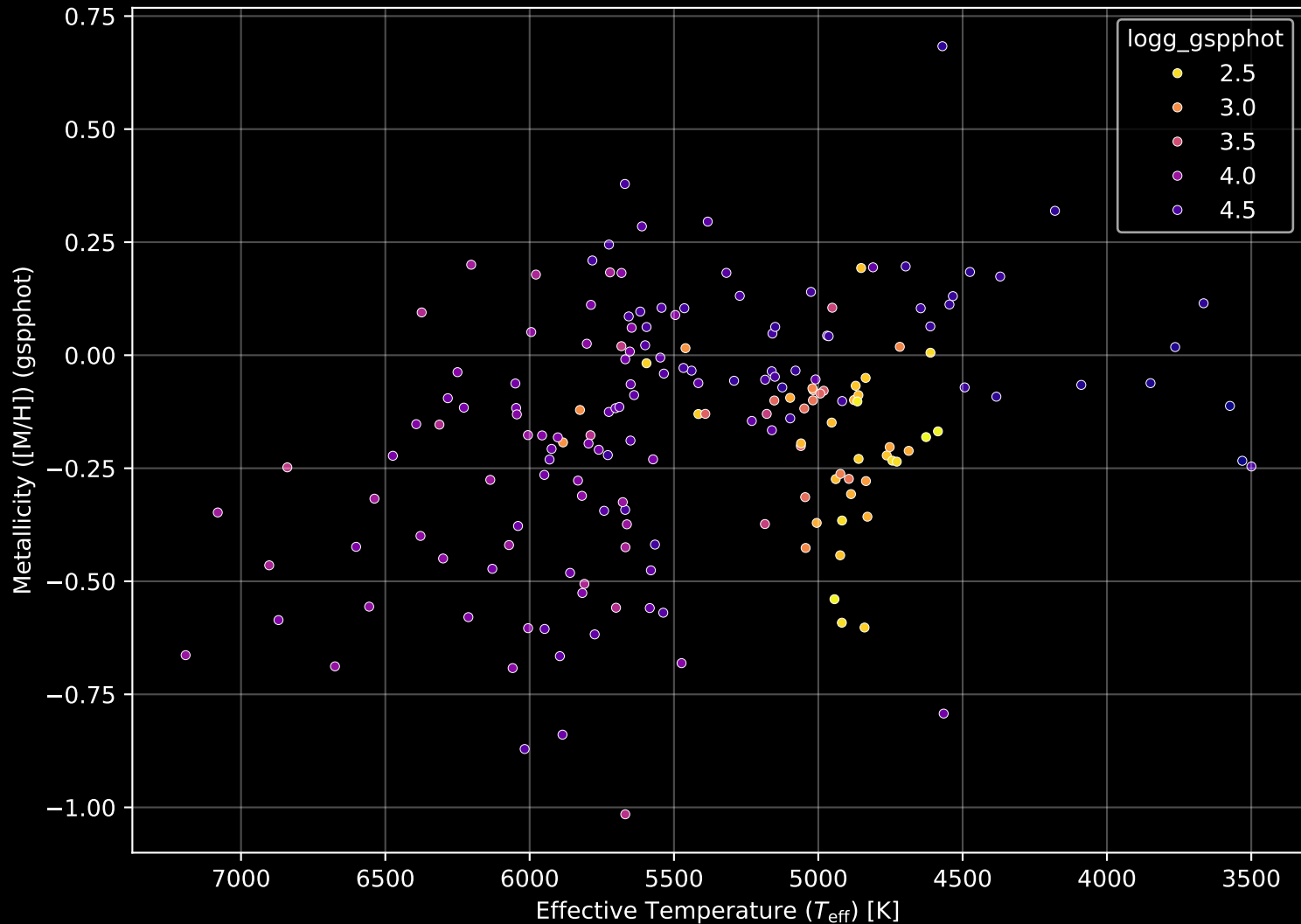
APOGEE DR17 Field: [063+47_MGA] Stellar Population Parameters (n= 183)
